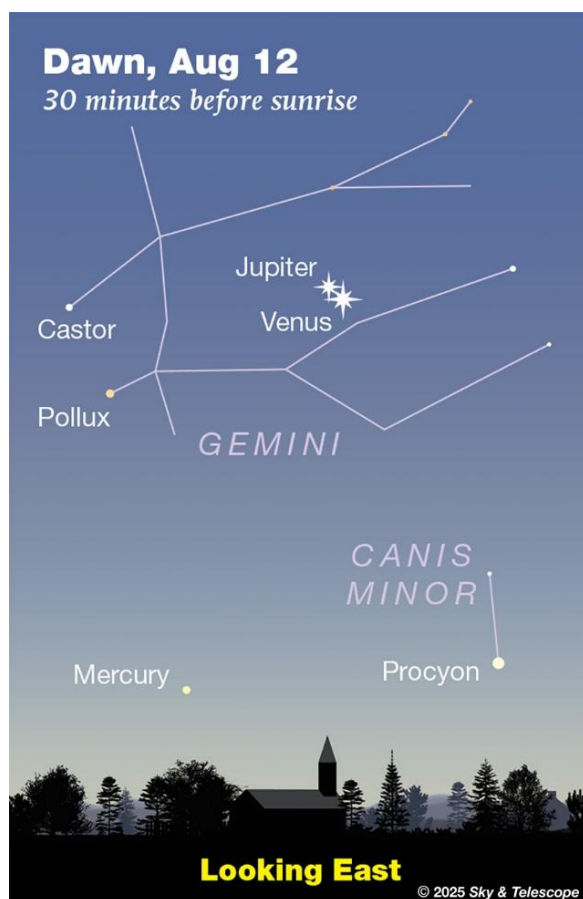
Congiunzione Venere-Giove all'alba del 12 agosto 2025 (da Sky & Telescope).
