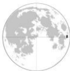
N. Mare Spumans (Sea of Foam)
